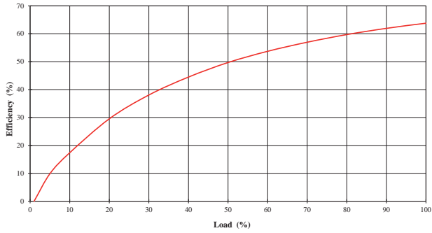
MGJ1D051905MPC
