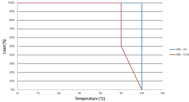
MGJ1D051505MPC
