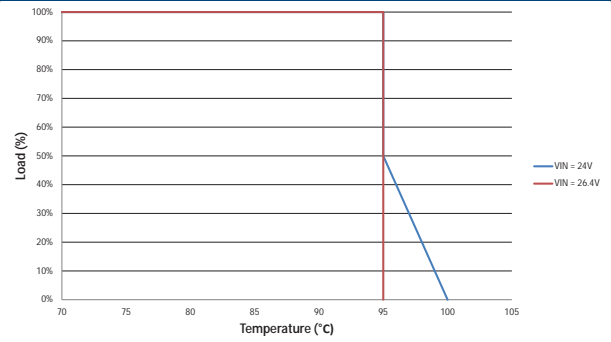
MGJ1D241905MPC
