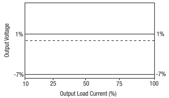
121505, 241505
