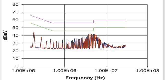
MGJ1D121505MPC
