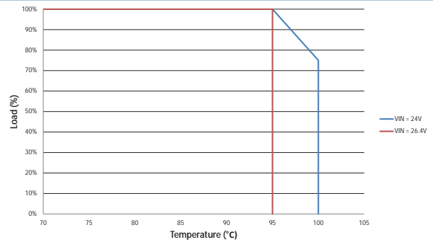
MGJ1D241505MPC
