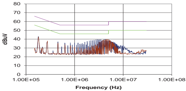
MGJ1D121509MPC
