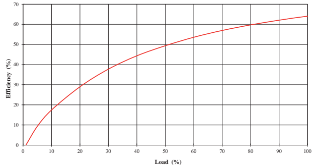
MGJ1D121505MPC
