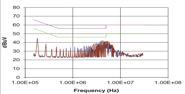
MGJ1D121905MPC
