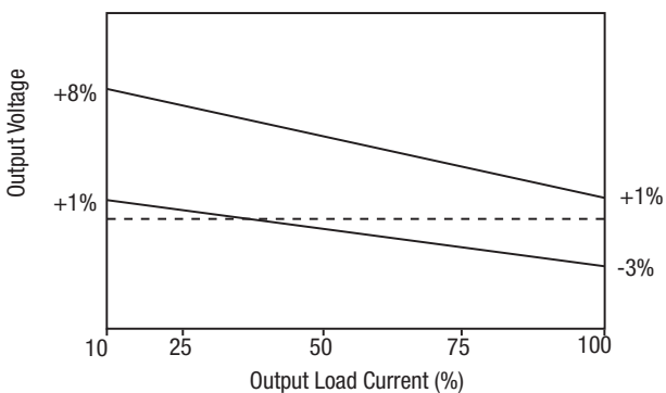
15V Output
