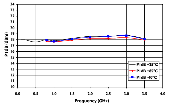
P1dB
