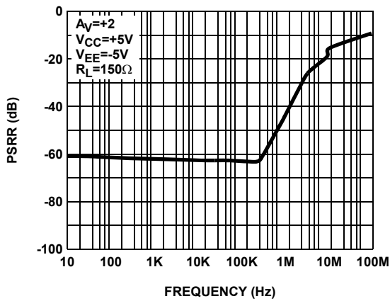
FIGURE 13. PSRR (V EE )
