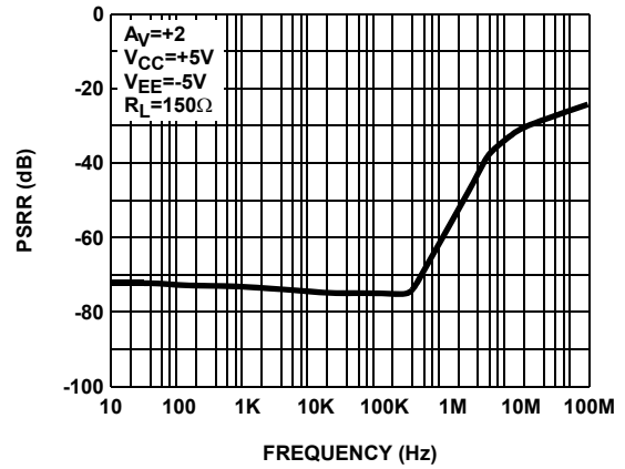
FIGURE 12. PSRR (V CC )
