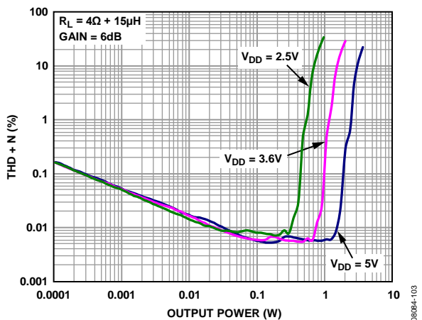
Figure 5. THD + N vs. Output Power into 4Ω, Av = 6 dB
