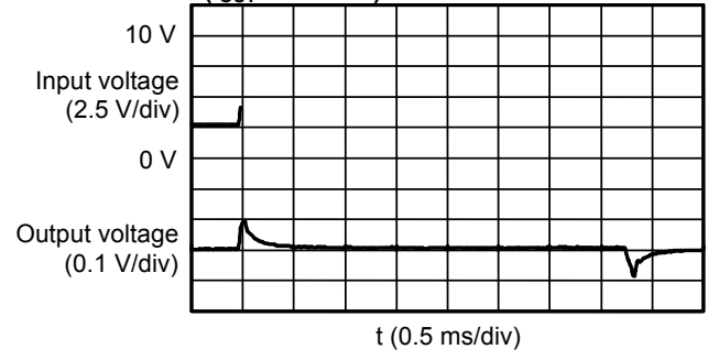
S-8533A15AFT ( I_{OUT} : 500 mA)
