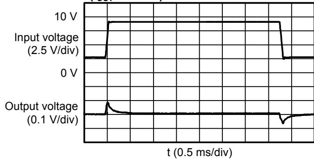
S-8533A15AFT ( I_{OUT} : 10 mA)
