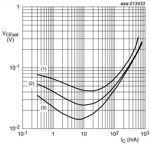
T_{amb} = 25\text{ }^\circ\text{C} (1) I_C/I_B = 10 (2) I_C/I_B = 5 (3) I_C/I_B = 2.5
