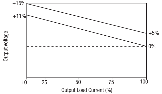
NXE2S1215MC
