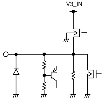
11pin<CPUSB#>
