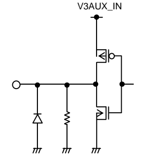
12pin<CPPE#>
