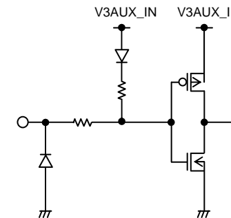
8pin<PERST#>
