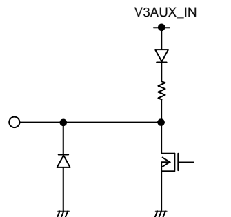
19pin<RCLKEN >
