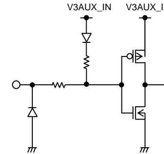
17pin<V3AUX>
