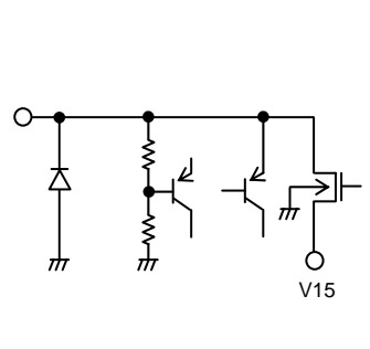
15,16pin<V15_IN1,V15_IN2>
